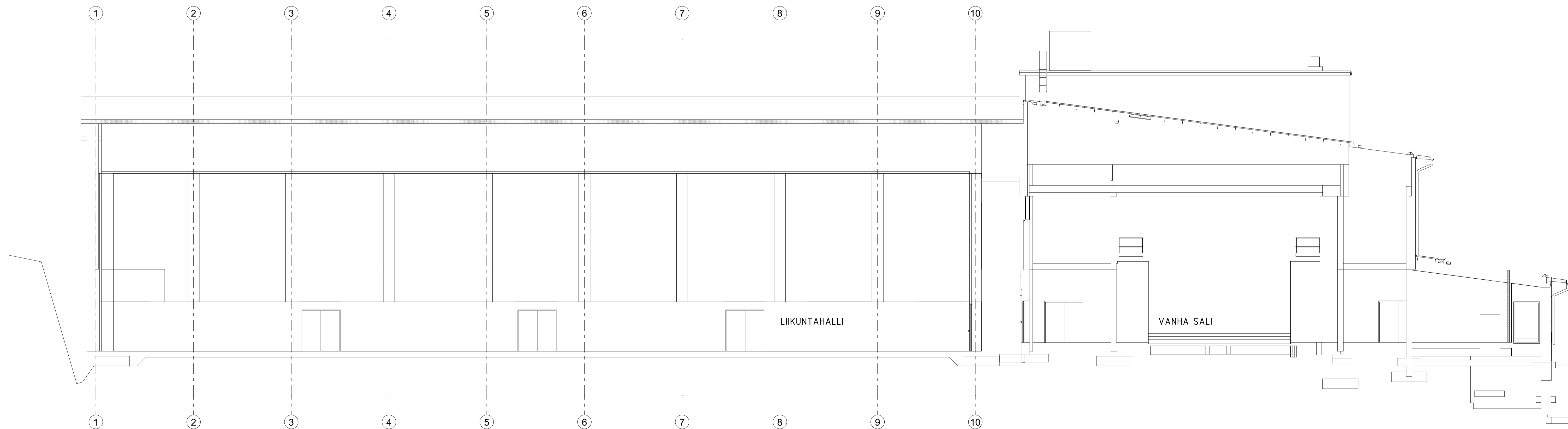
LEIKKAUS D-D
