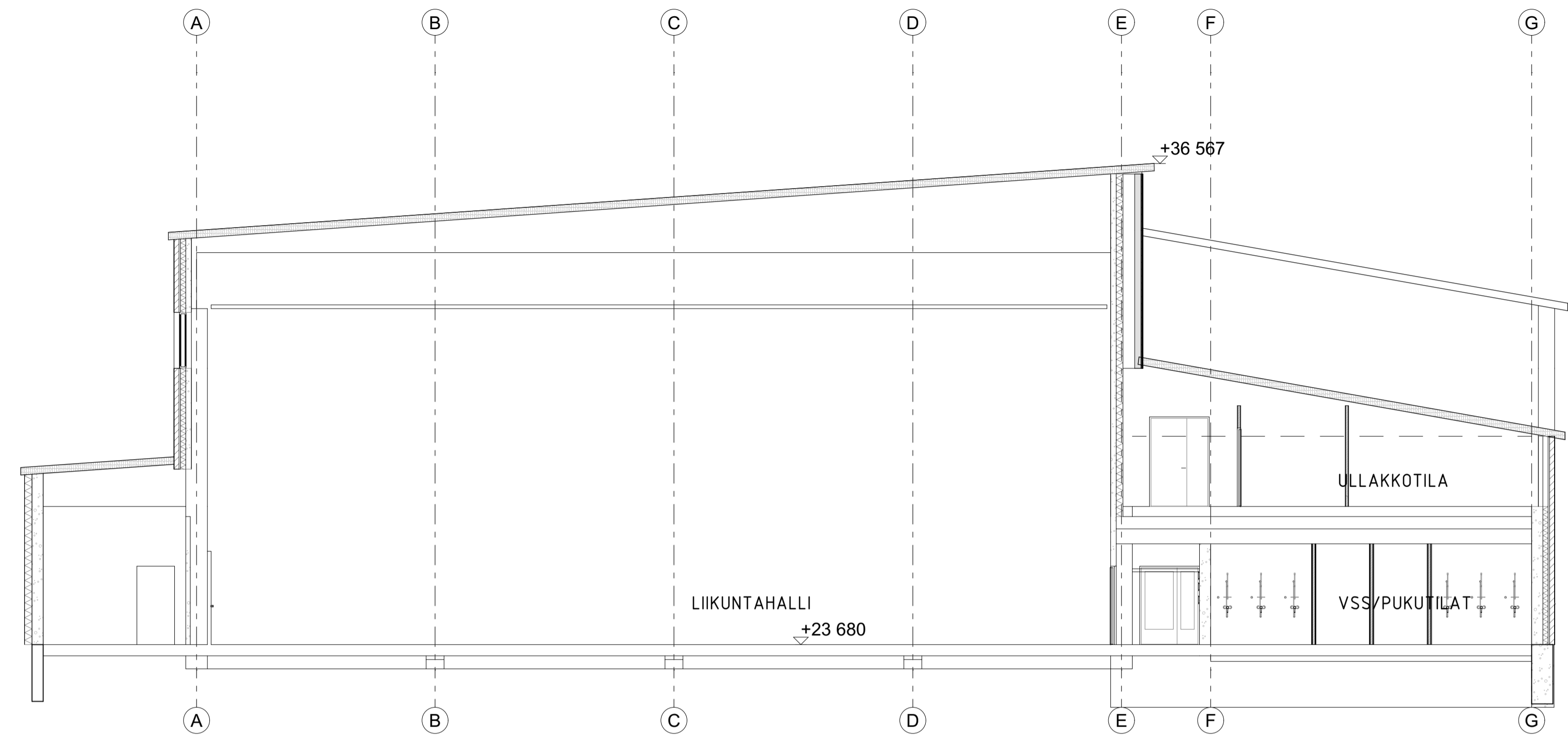
LEIKKAUS B-B
