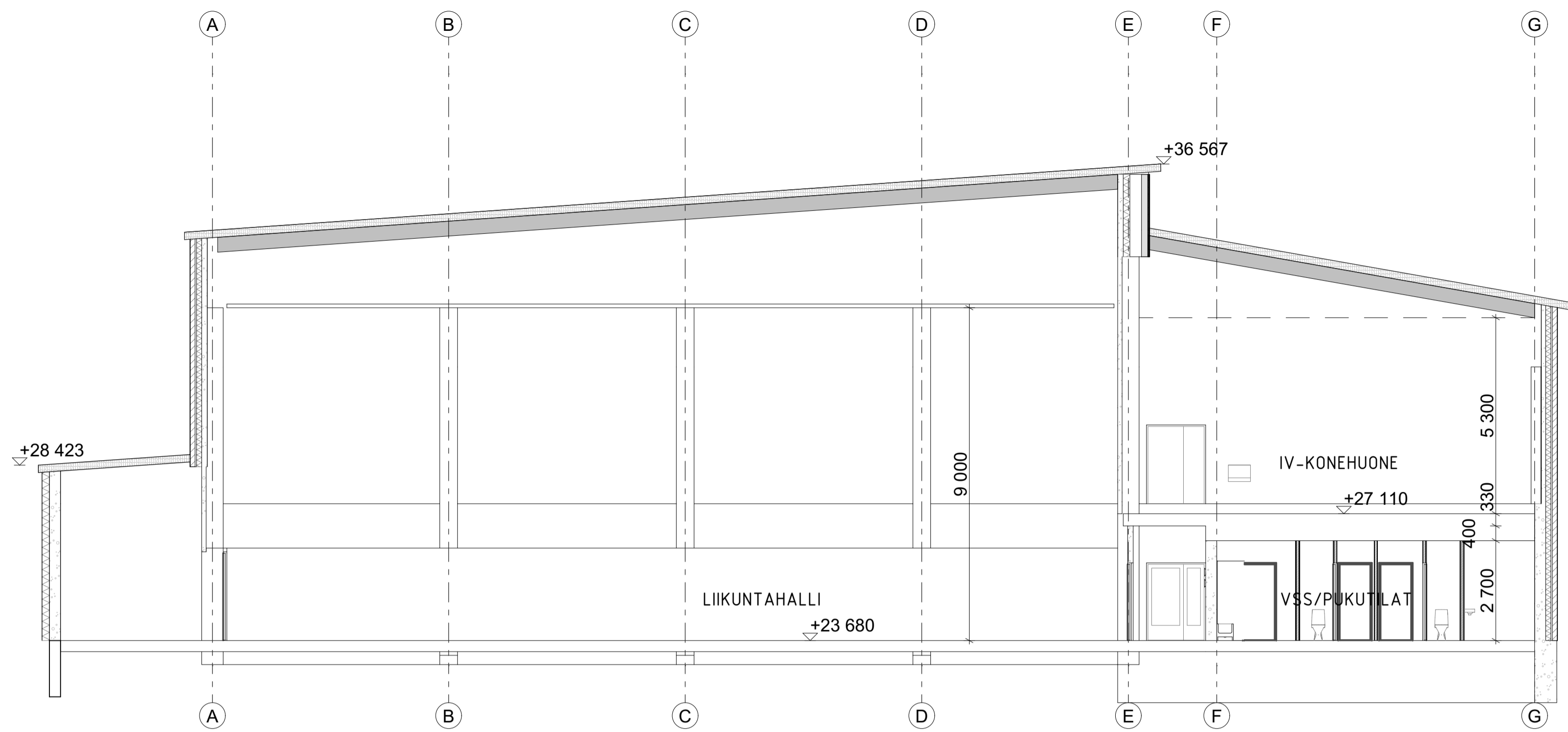
LEIKKAUS A-A
