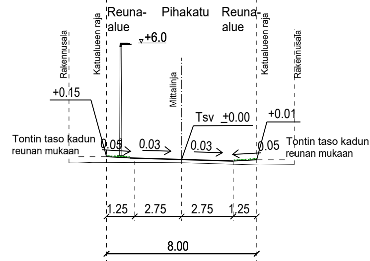
TYYPPIPOIKKILEIKKAUS MATILDANPOLKU PL 20 1:200
