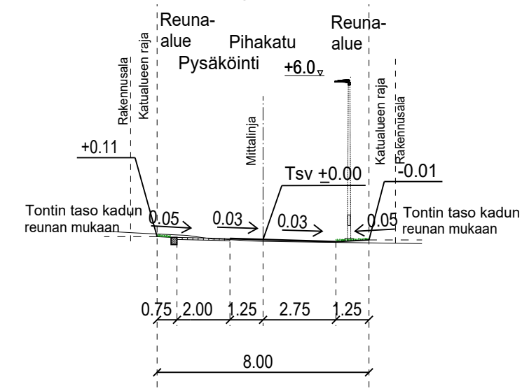
TYYPPIPOIKKILEIKKAUS MÄNTYPELLONTIE PL 380 1:200
