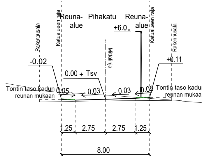
TYYPPIPOIKKILEIKKAUS MÄNTYPELLONTIE PL 240 1:200
