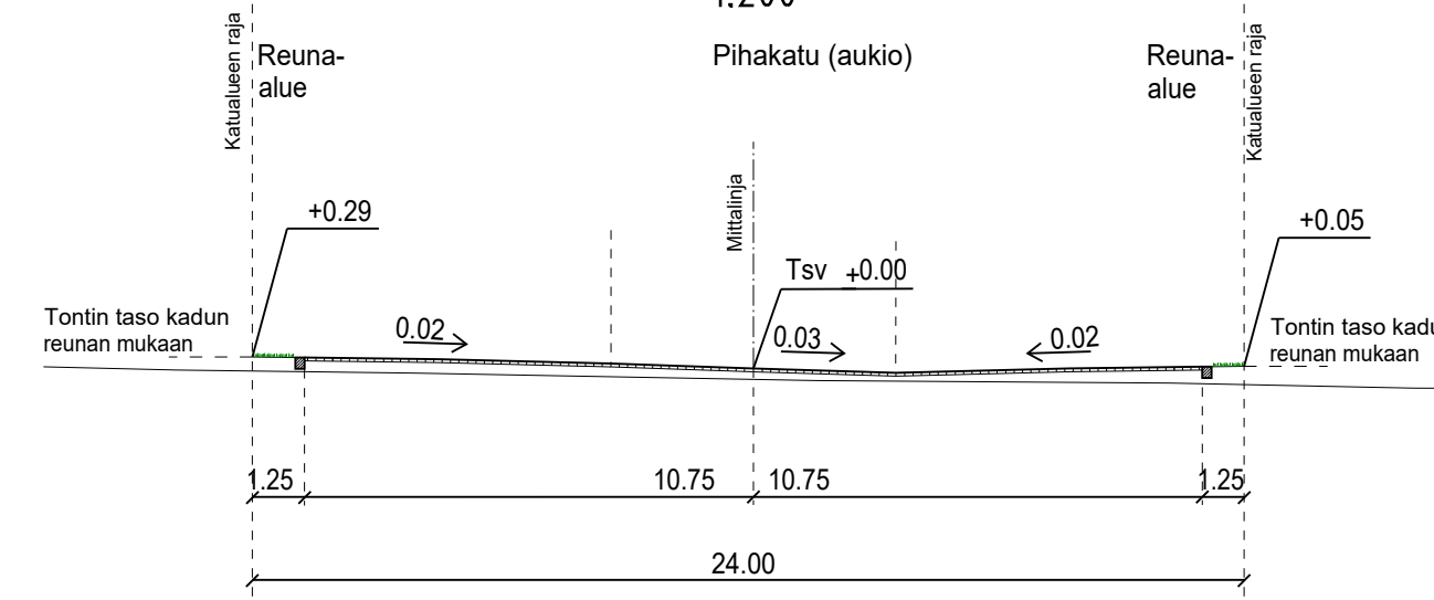
TYYPPIPOIKKILEIKKAUS MÄNTYPELLONTIE PL 330 1:200
