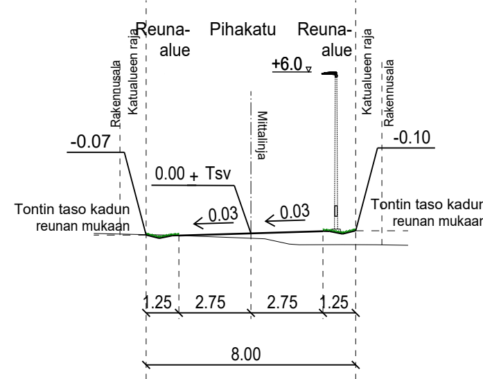
TYYPPIPOIKKILEIKKAUS RIIHIMÄENTIE PL 120 1:200
