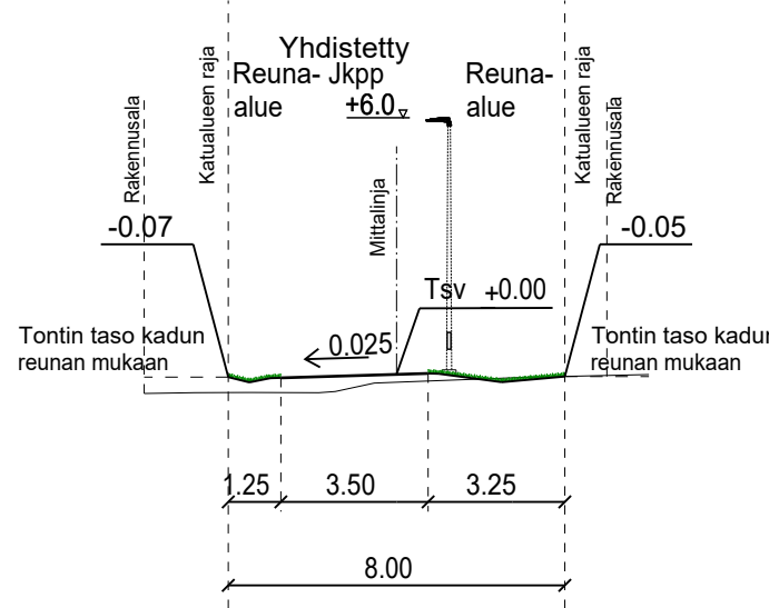
TYYPPIPOIKKILEIKKAUS RIIHIMÄENTIE PL 20 1:200
