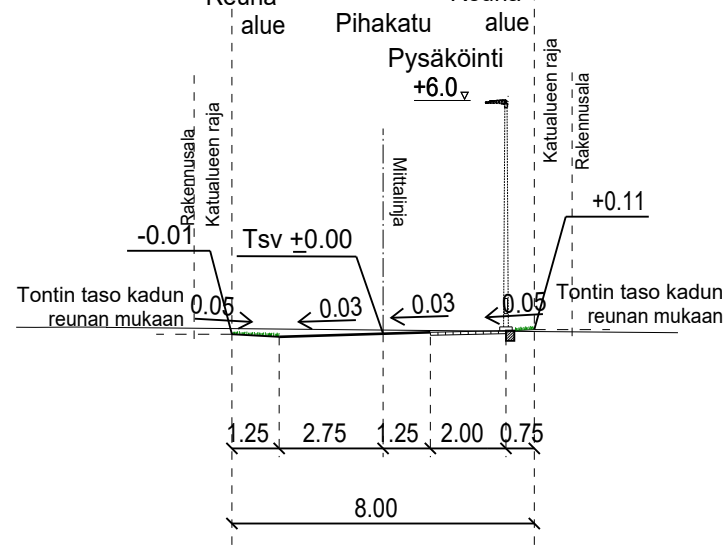
TYYPPIPOIKKILEIKKAUS RIIHIMÄENTIE PL 50 1:200
