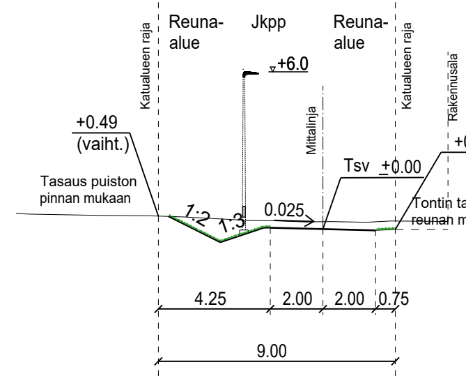
TYYPPIPOIKKILEIKKAUS POHJANMETSÄNREUNA PL 80 1:200
